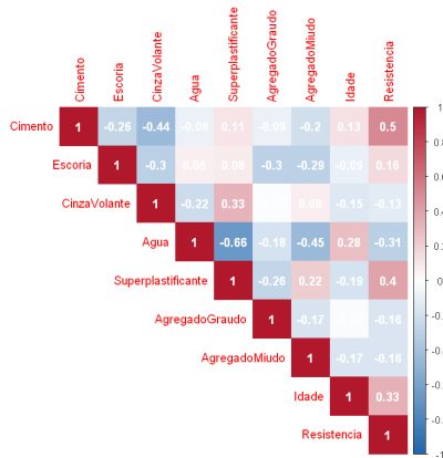
Figura 2: Corrplot das variáveis numéricas
